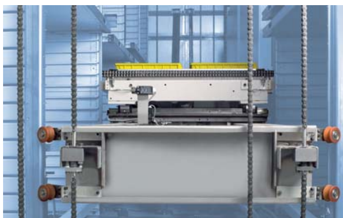
Système à 4 chaînes pour un guidage parfait de l'extracteur
