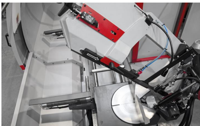
Vérin de descente et palpeur approche rapide archet
